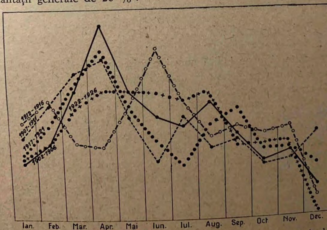
Fig. 14. — Curbele procentuale ale frecvenței nașterilor în diferite luni ale anului pentru grupele de ani: 1902—1906 1907—1911 1912—1916 1917—1921 1922—1926.
