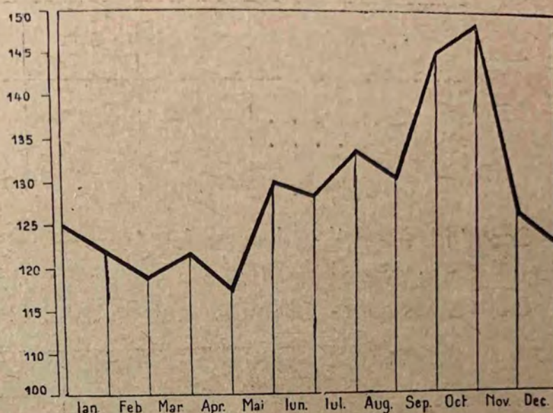
Fig. 13. — Natalitatea lunară în comuna Drăguș-Făgăraș
