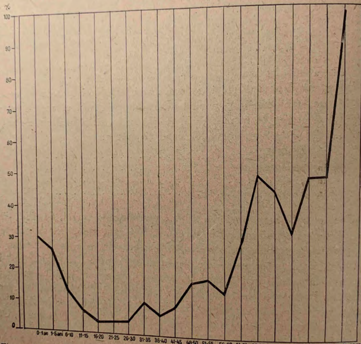
Fig. 5.—Mortalitatea bărbaților din neamul Fogoros (Drăguș) calculată în decursul unui secol.
