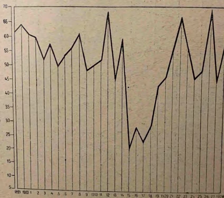
Fig. 11. — Nașterile dela 1899—1928 în Drăguș
