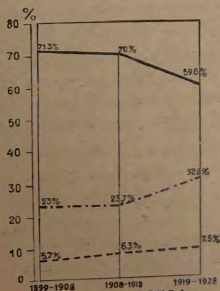
Fig. 10. — Diferențe de vârstă la căsătorii în Drăguș.
